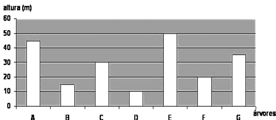
Altura de algumas árvores brasileiras
